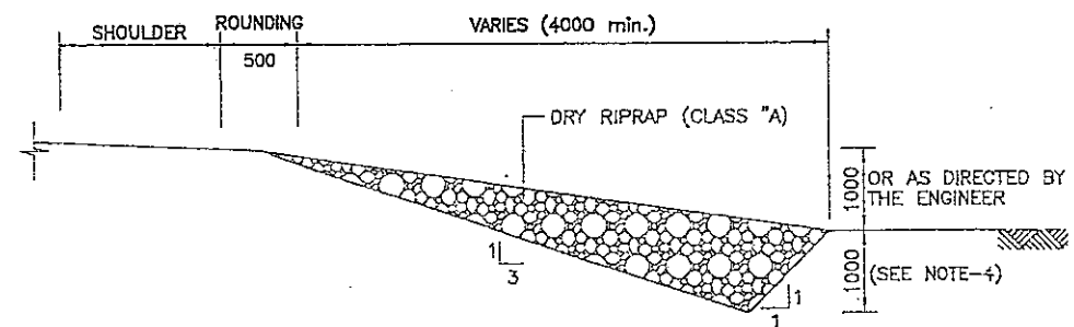
DRY RIPRAP PROTECTION (EP-2)
